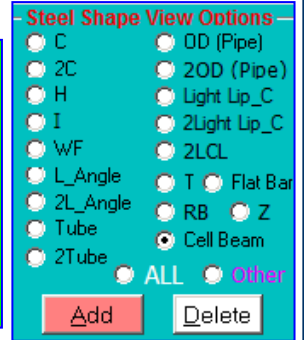
ต.ย. หน้าตัด Cellular Beam ในตารางเหล็ก MicroFeap 6.2
